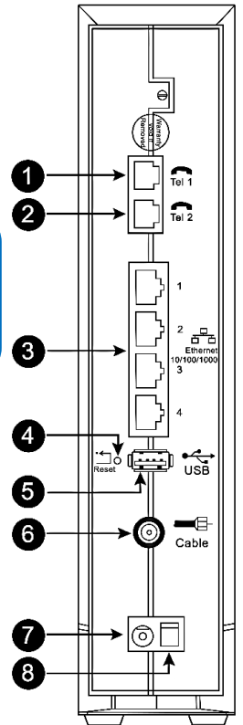
Kuva 1, liitännät
